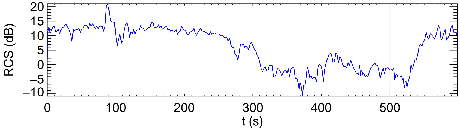
Ku-band RCS
